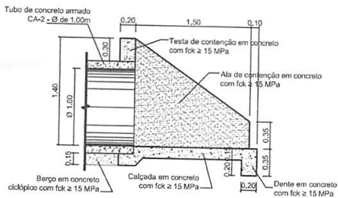
VISTA LATERAL
