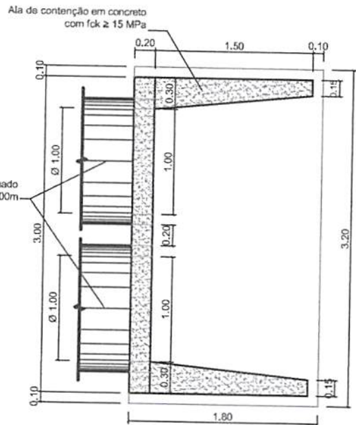
PLANTA BAIXA
