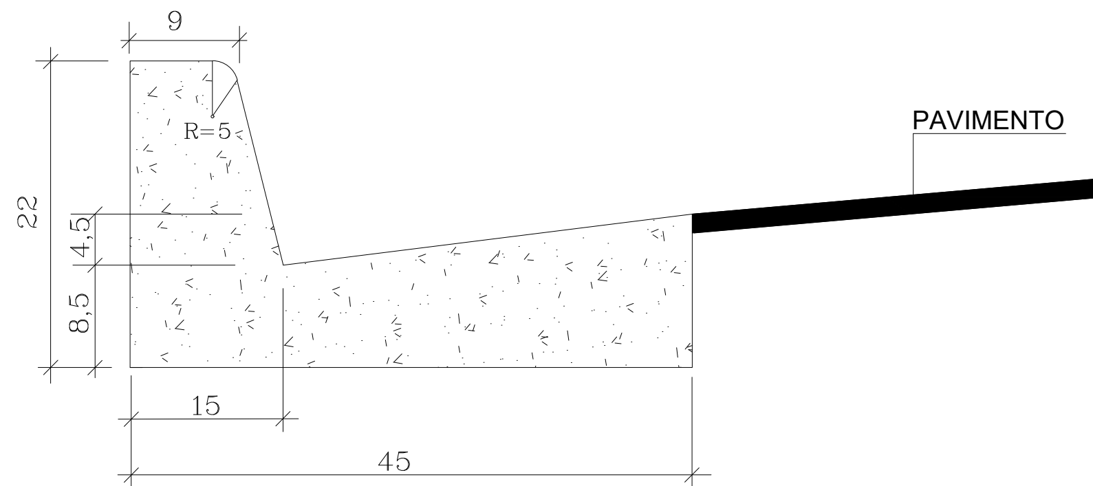
DETALHE DO MEIO FIO E SARJETA
