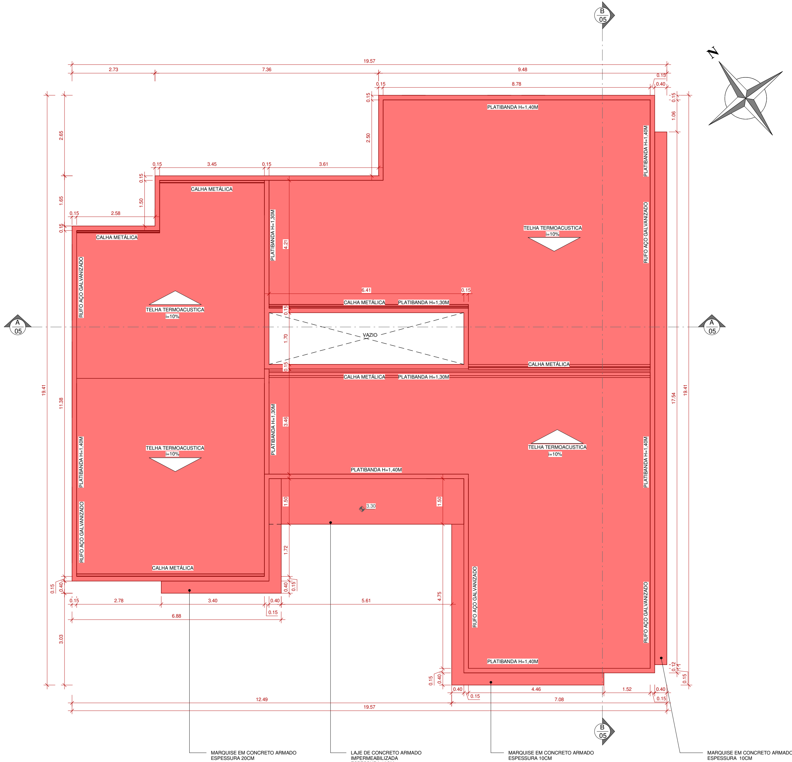
2 PLANTA DE COBERTURA - CONSTRUIR 1 : 75
