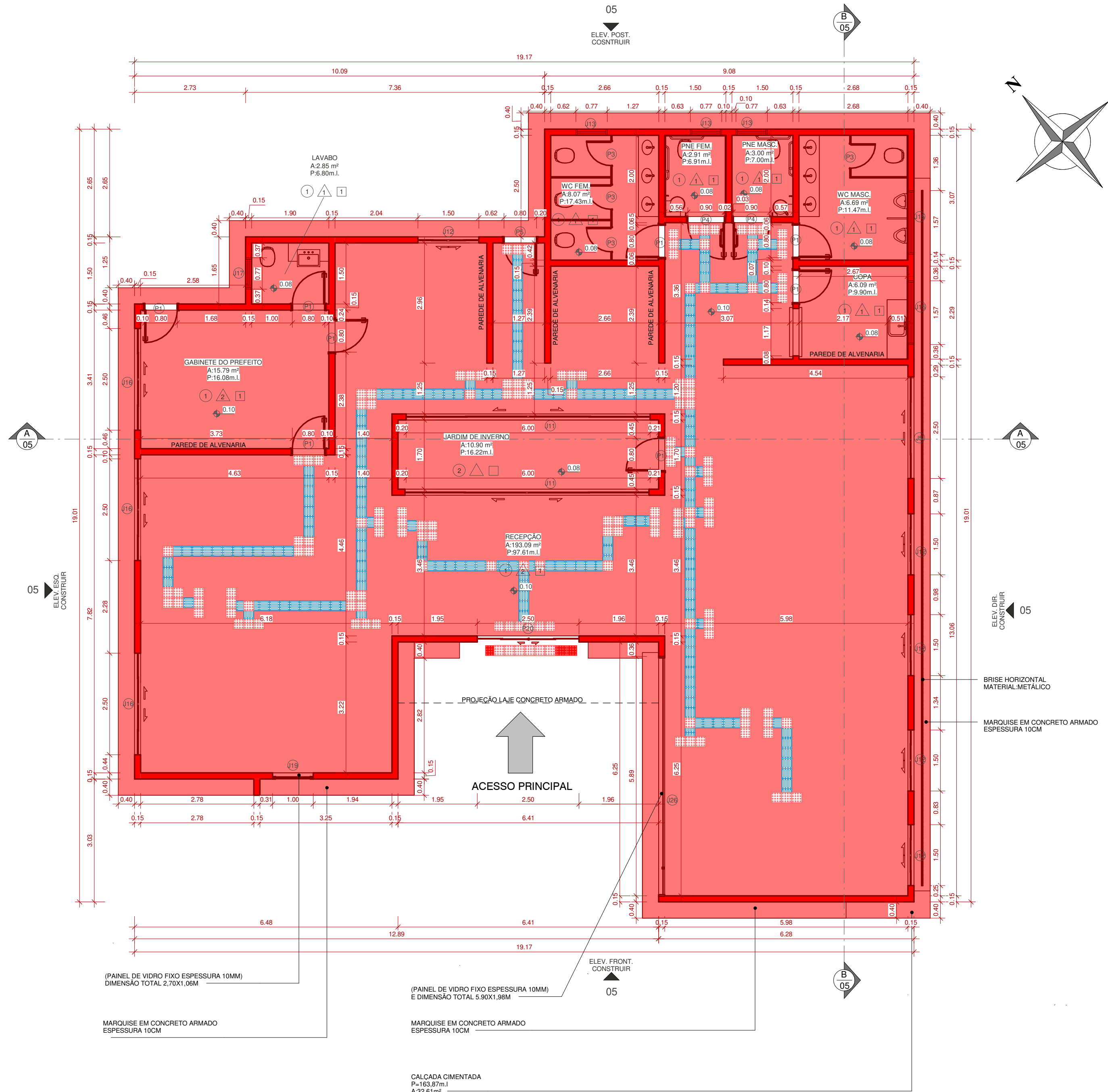
1 PLANTA BAIXA-CONSTRUIR 1 : 75
