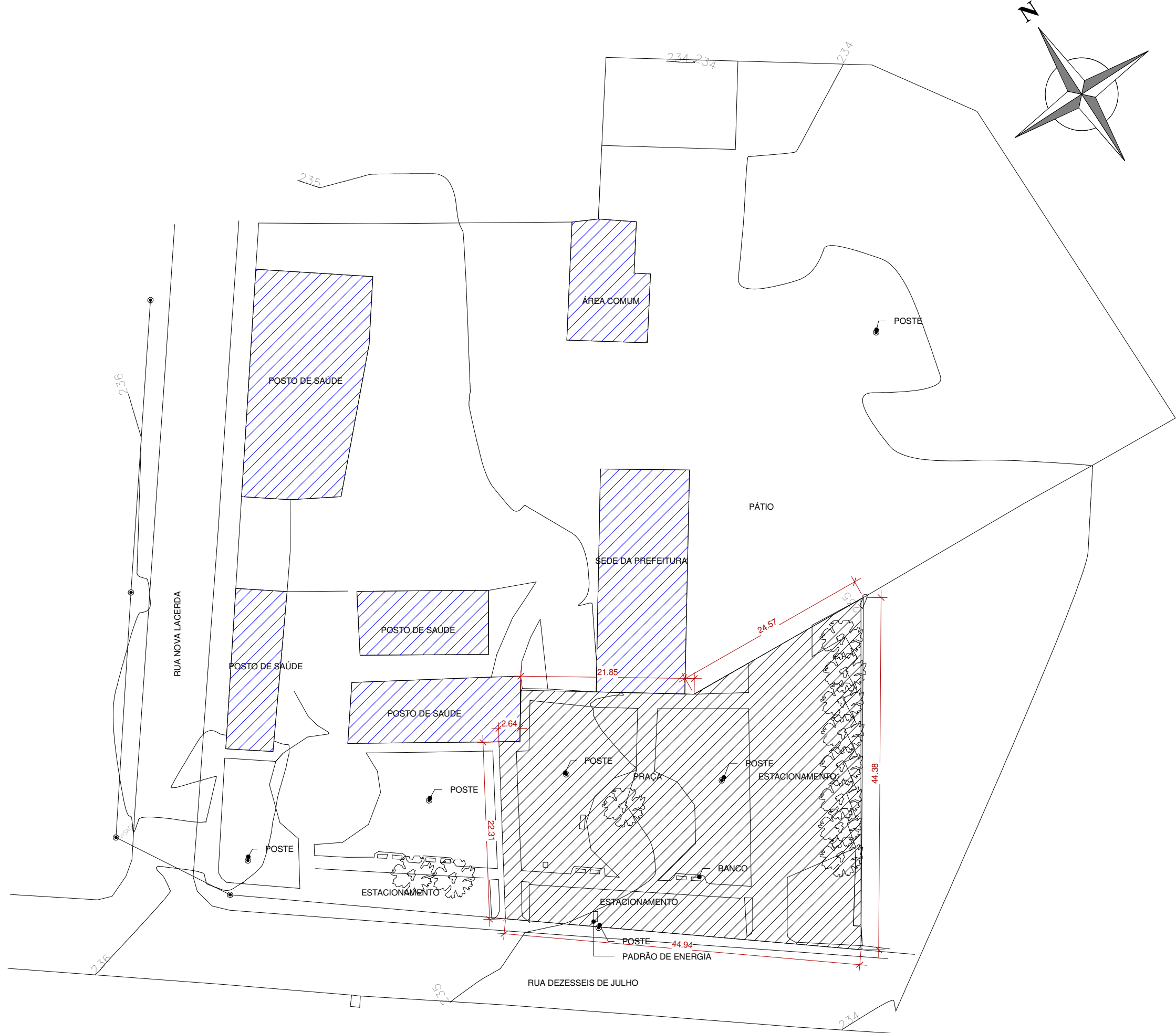
PLANIALTIMÉTRICO/CROQUI DO TERRENO 1 : 500
