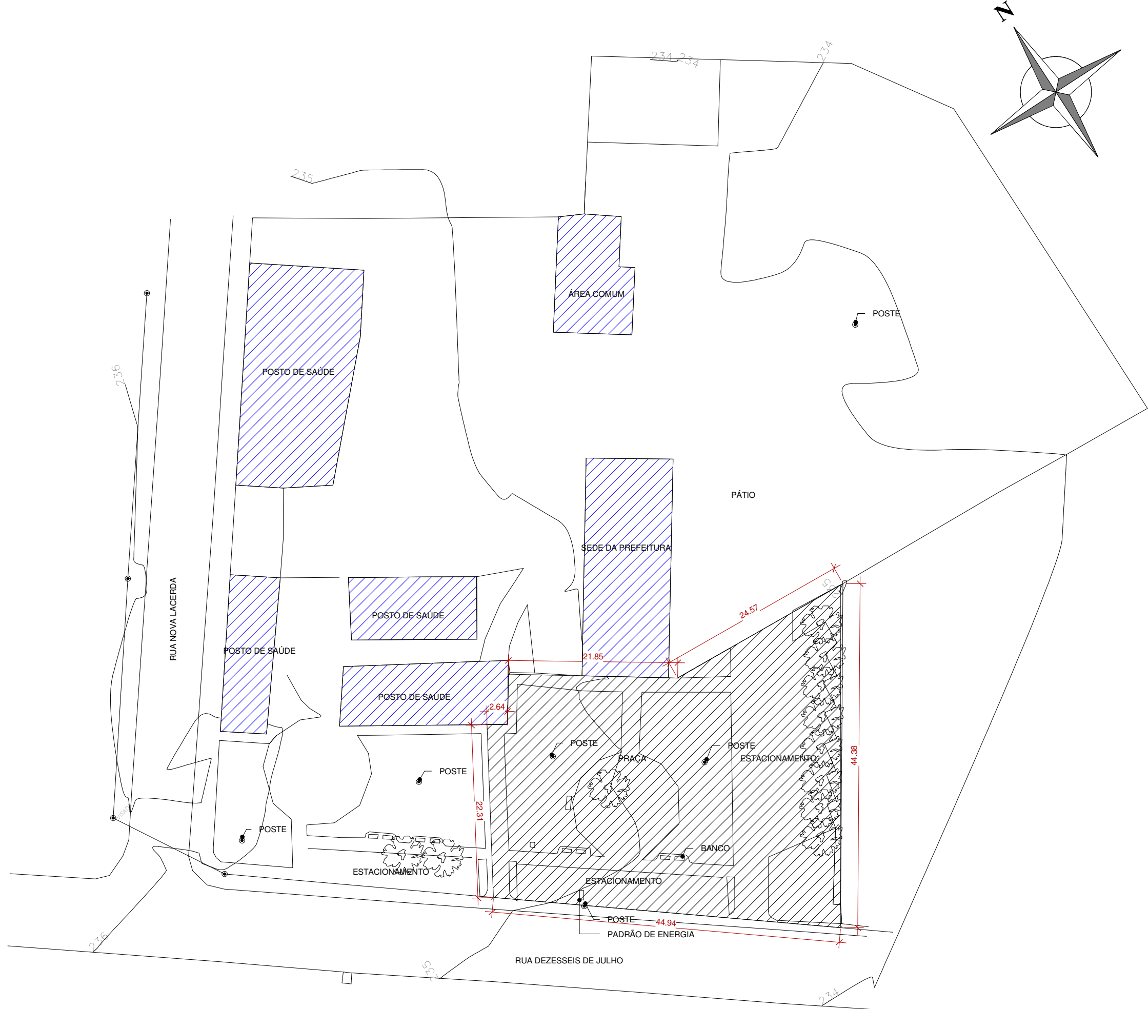
PLANALTIMÉTRICO/SITUAÇÃO 1 : 500
