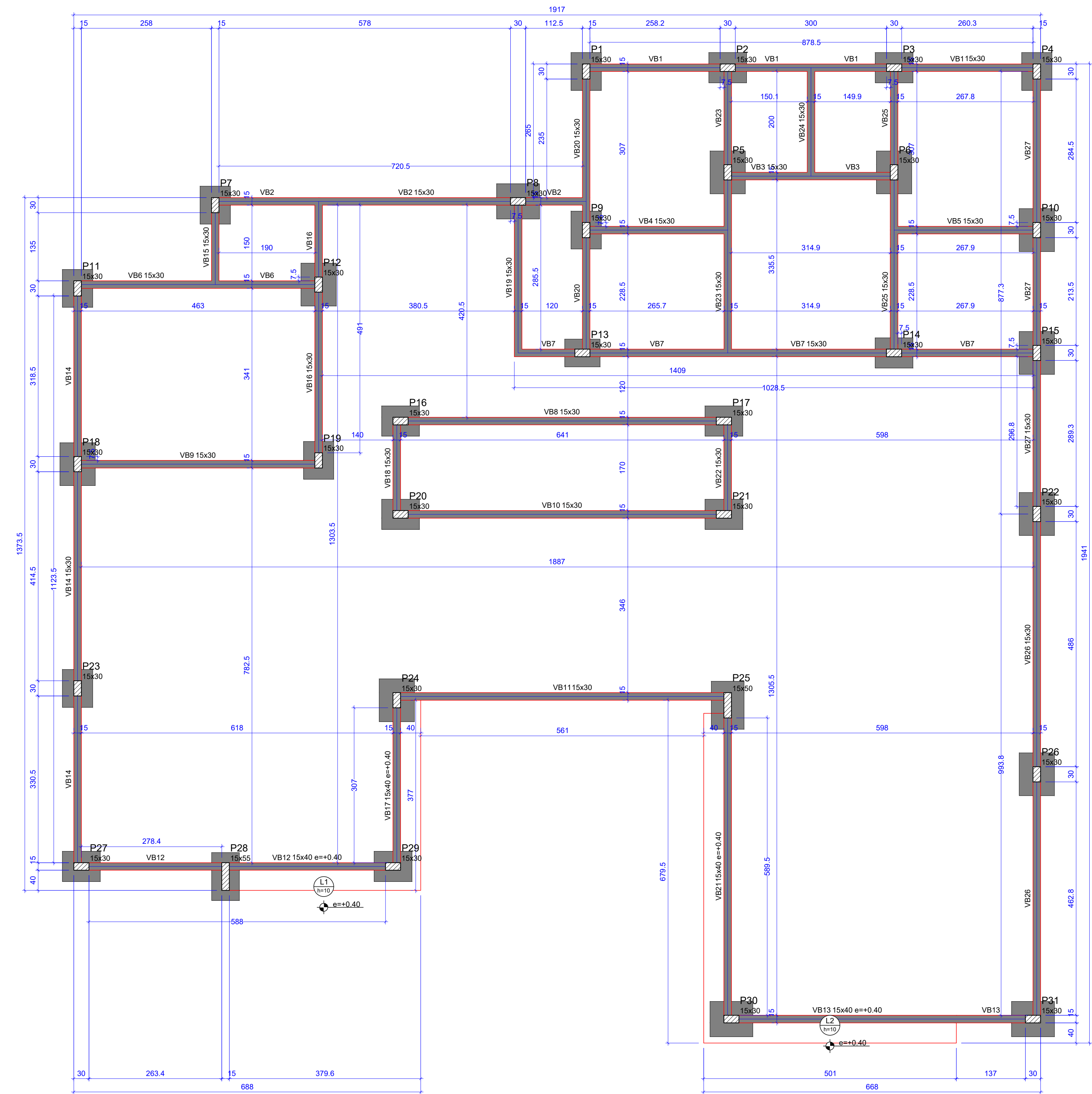
Forma do pavimento Baldrame (Nível 0.00) escala 1:50
