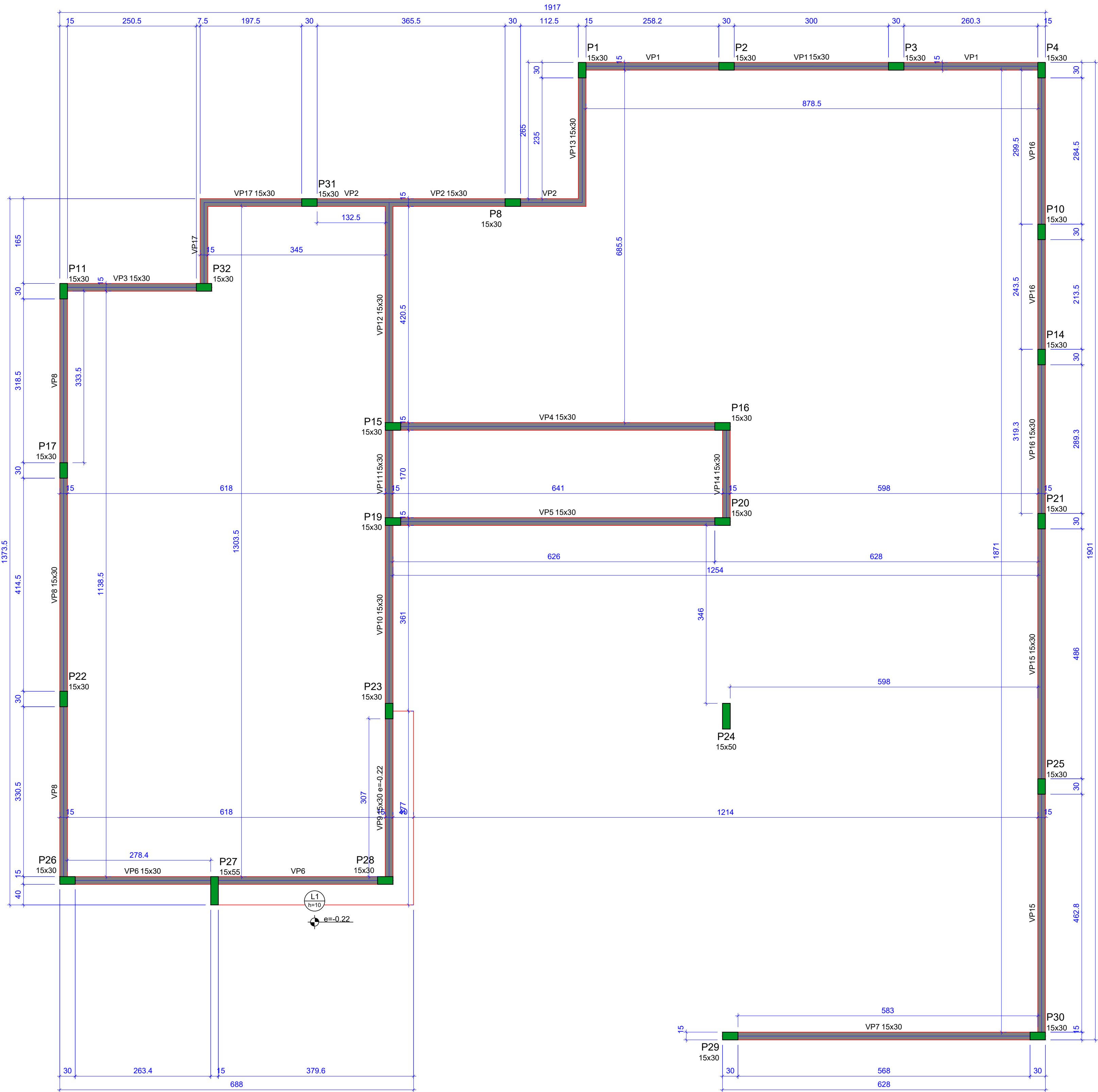
Forma do pavimento Platibanda (Nível 4.50) escala 1:50
