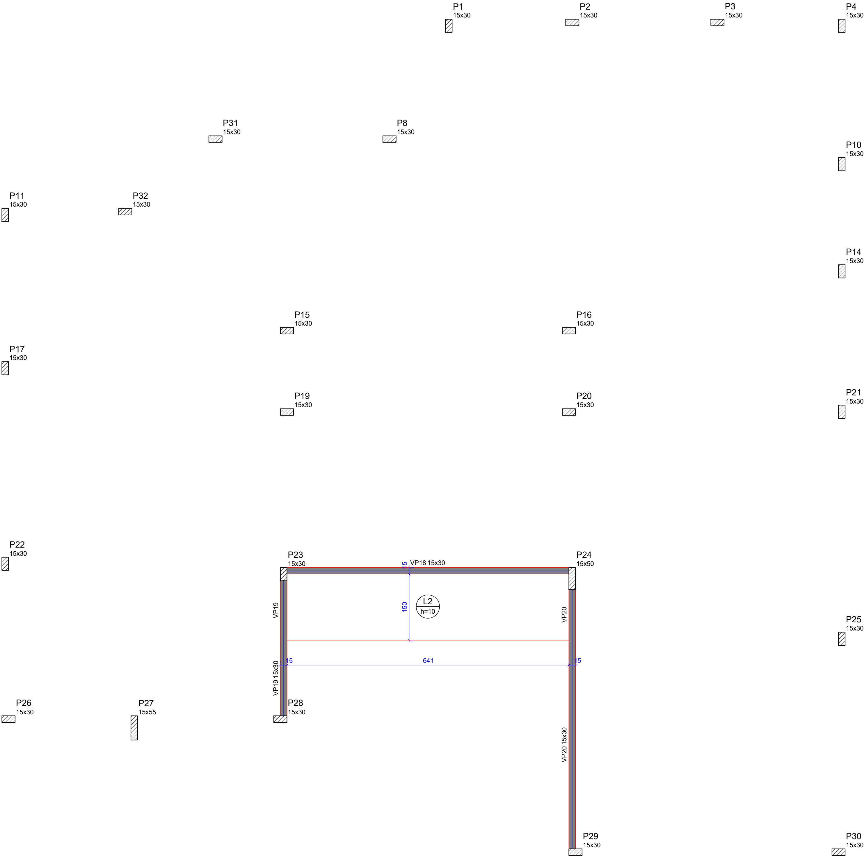
Forma intermediária do pavimento Platibanda (Nível 3.50) escala 1:50
