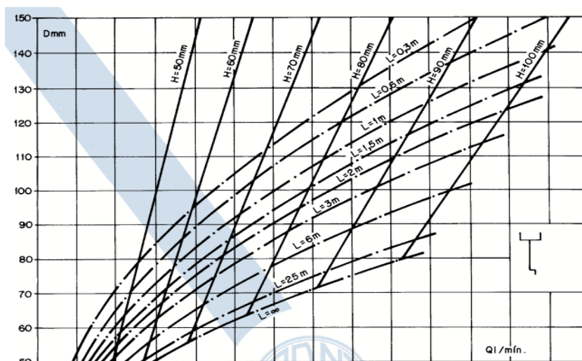
Ábaco 1: Ábaco para determinação de diâmetros de condutores verticais. Fonte: NBR 10844/89
