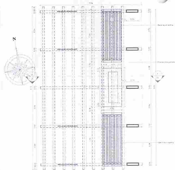
3 PLANTA BAIXA ESTÁÇÕES DE CONTEMPLAÇÃO Escala: 1 : 30
